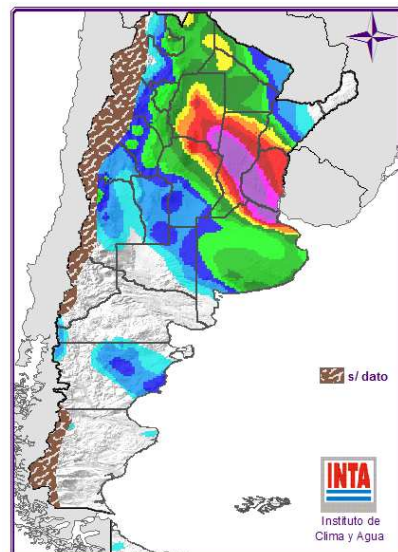
Fig. : Precipitación pronosticada (mm) entre el 30 de octubre y el 2 de noviembre de 2013, entre las 9 hs del día del pronóstico y las 9 hs del día siguiente.
